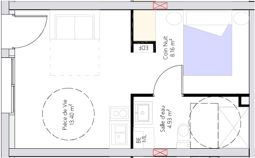
LOGEMENT 08 VUE EN PLAN - Ech. 1/75
