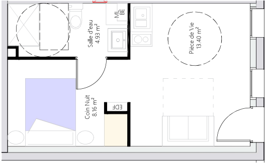
LOGEMENT 06 VUE EN PLAN - Ech. 1/75
