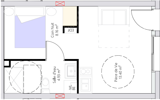
LOGEMENT 05 VUE EN PLAN - Ech. 1/75
