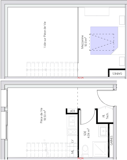
LOGEMENT 24 VUE EN PLAN - Ech. 1/75
