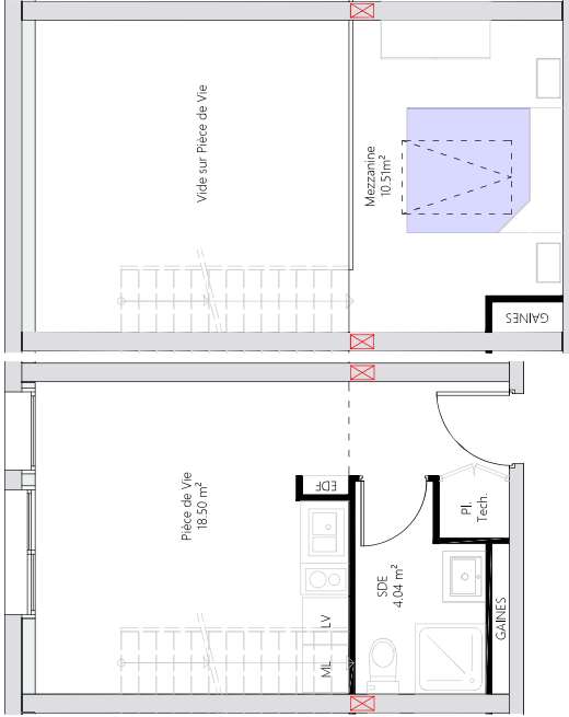
LOGEMENT 20 VUE EN PLAN - Ech. 1/75
