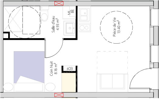
LOGEMENT 02 VUE EN PLAN - Ech. 1/75
