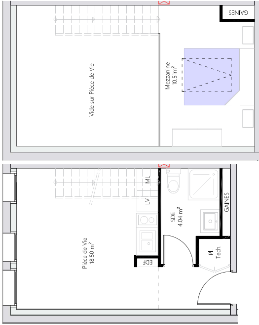
LOGEMENT 19 VUE EN PLAN - Ech. 1/75
