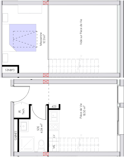
LOGEMENT 17 VUE EN PLAN - Ech. 1/75
