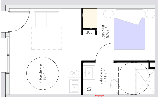
LOGEMENT 12 VUE EN PLAN - Ech. 1/75
