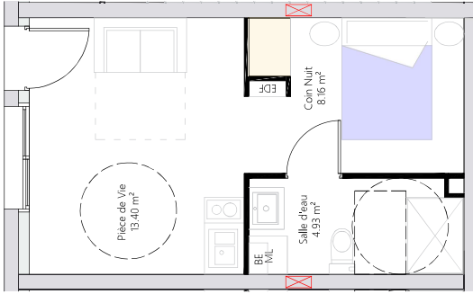
LOGEMENT 10 VUE EN PLAN - Ech. 1/75
