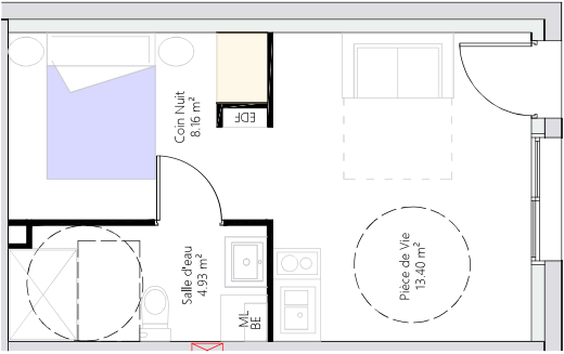
LOGEMENT 01 VUE EN PLAN - Ech. 1/75
